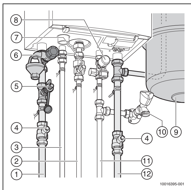
Afb. 2 Overzicht aansluitingen
