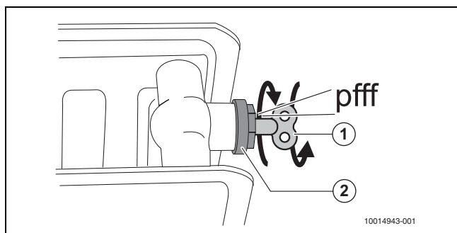
Afb. 8 Ontluchten radiator
