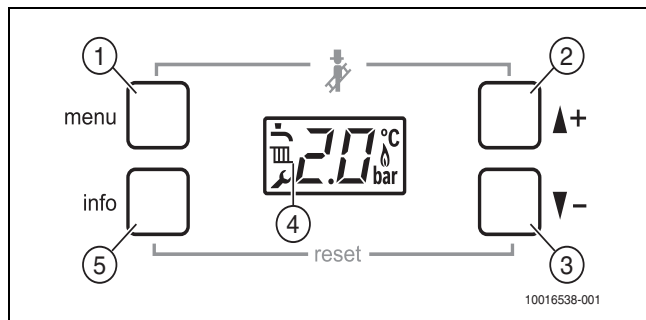
Afb. 6 Bedieningspaneel
